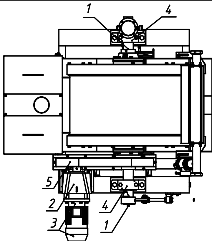
Рис.6. Расположение точек смазки
