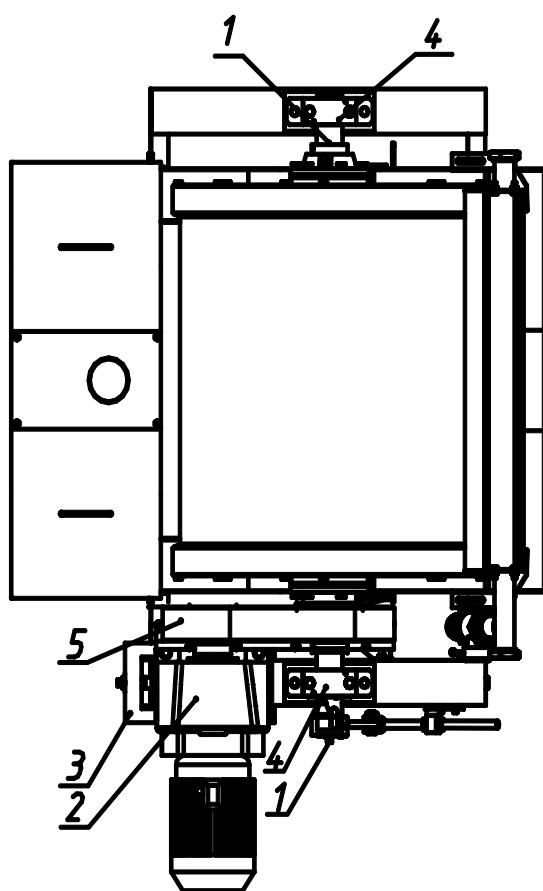
Рис.6. Расположение точек смазки
